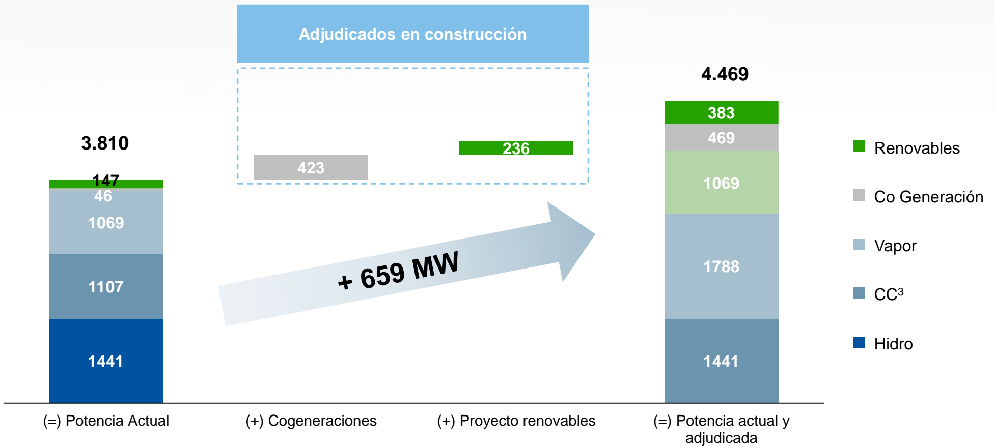
Activos de generación actuales y en construcción por tecnología (MW) 1
